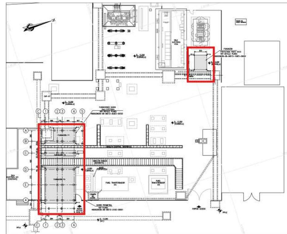
Figura 4-5 – Emplazamiento de Nueva Sala Eléctrica N°2
